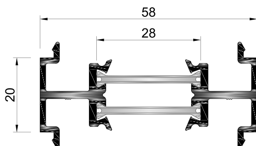
LT.37 Perfil Ligação
