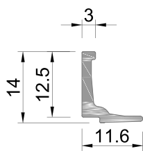
LT.905 Brite Folha Oculta (Poliamida)
