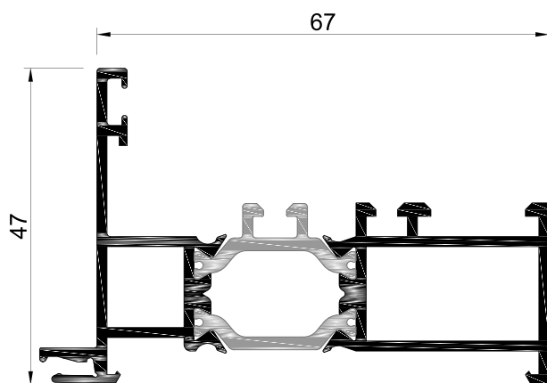
LT.31 Aro Fixo
