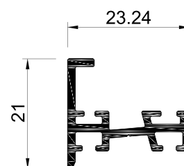
IT.33 Bite Inferior de Vedação
