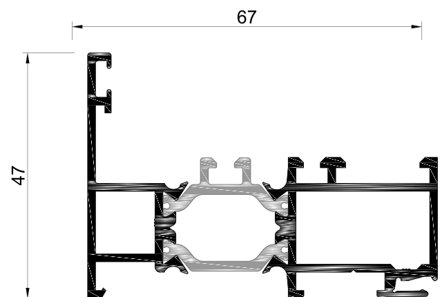
LT.41 Aro Fixo
