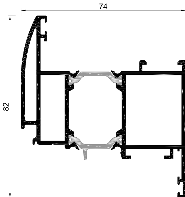
LT.88 Aro Móvel
