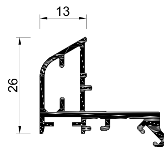
LT.32 Bite Inferior de Vedação
