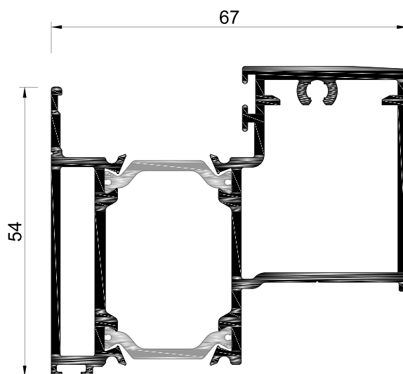
LT.92 Aro Móvel Folha Oculta - Portas
