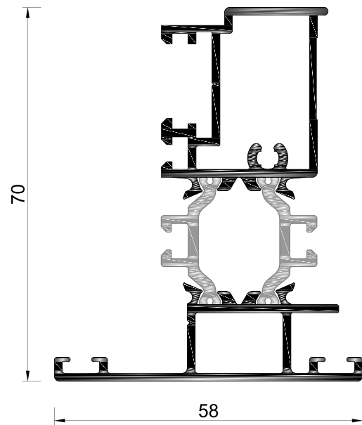
LT.96 Inversor Oculta
