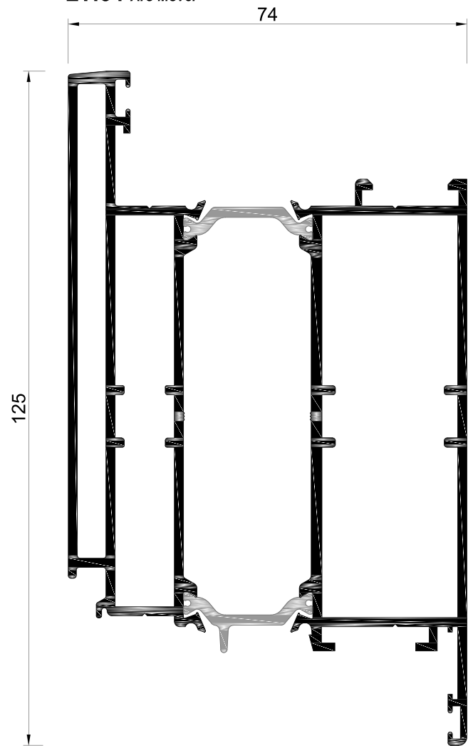
LT.64 Aro Móvel
