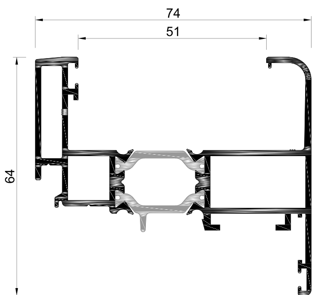
LT.03 Aro Móvel
