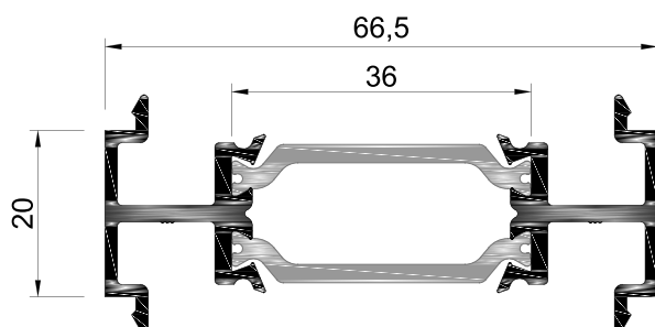
LT.35 Perfil Ligação
