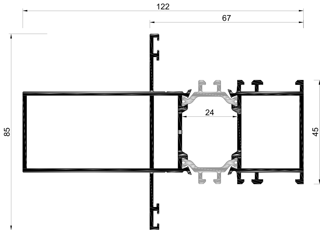
LT.19 Montante
