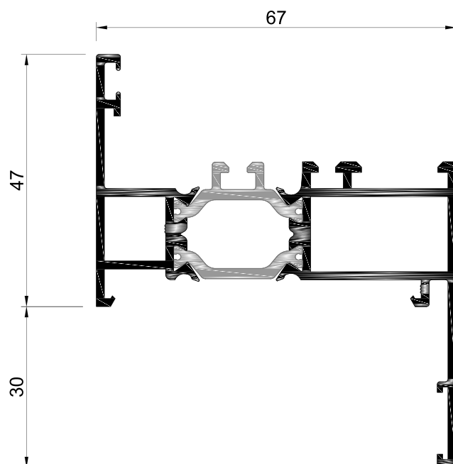
LT.61 Aro Fixo c/ Remate
