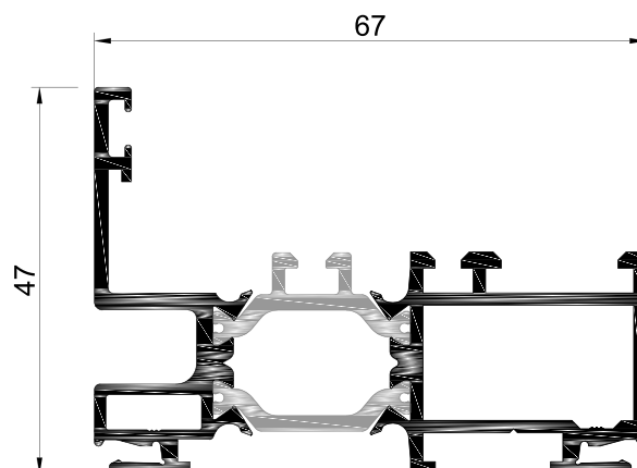
LT.71 Aro Fixo
