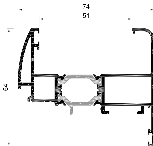
LT.63 Aro Móvel
