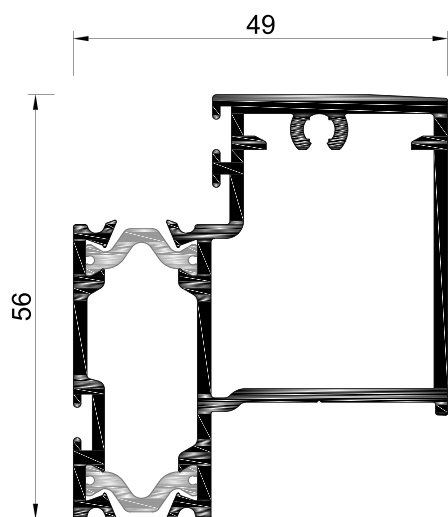
LT.91 Aro Móvel Folha Oculta - Portas
