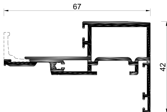
LT.90 Aro Móvel Folha Oculta
