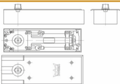
Mola de Pavimento para batente e vai-vem Peso máximo: 120Kg/folha
