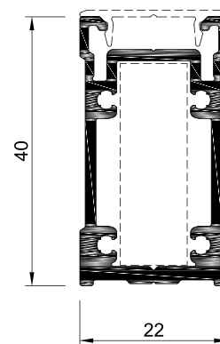
OS.25 Reforço / Puxador
