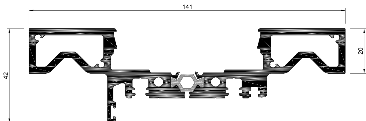
OS.58 Aro Móvel Lateral
