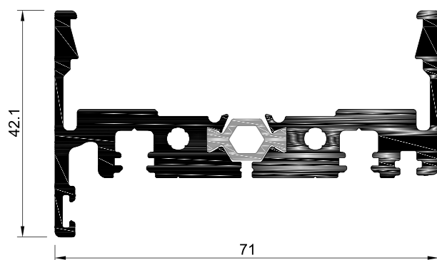
OS.76 Aro Móvel Lateral
