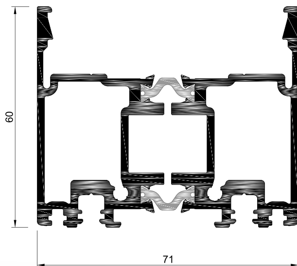
OS.69 Aro Móvel Sup./Inf.
