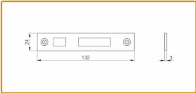
280010 TESTA SUP/INF 3x24 P/ FECHADURAS (Inox)
