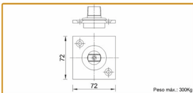
227114 PIVOT DE CHÃO 7471 AX
