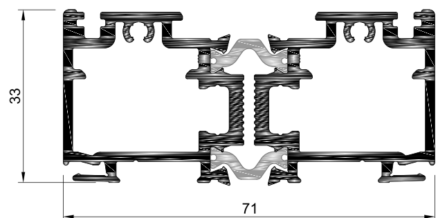
OS.80 Aro Fixo Superior
