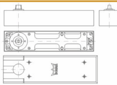
Mola de Pavimento para batente e vai-vem Peso máximo: 300Kg/folha
