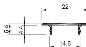
OS.30 Capa ( Aplicação no Perfil OS.25 )
