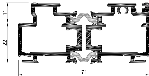
OS.78 Aro Fixo Lateral
