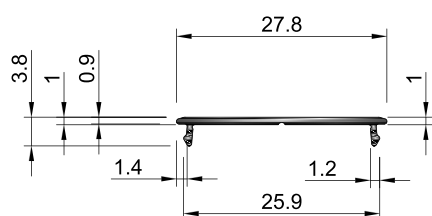
OS.906 Capa PVC ( Aplicação nos Perfis OS.78 e 80 )
