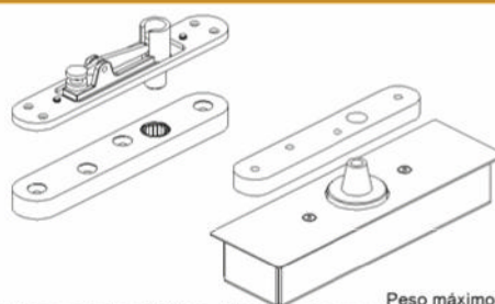
Peso máximo: 500Kg/folha Largura máxima por folha: 1500mm - Para larguras superiores, consultar Gab. Técnico
