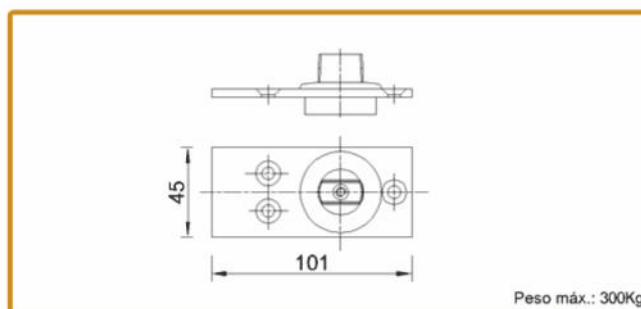
227115 PIVOT DE CHÃO 7475 AX
