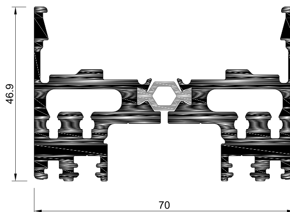
OS.74 Aro Móvel Sup./Inf.
