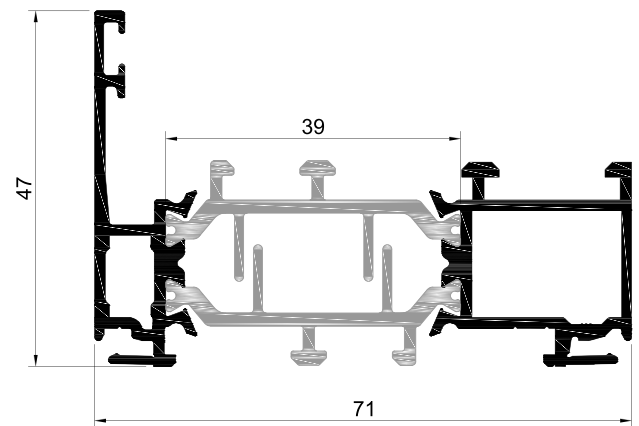
NST.51 Aro Fixo
