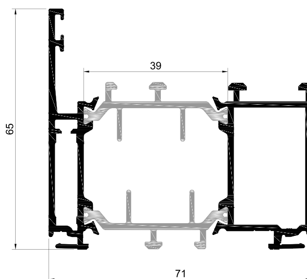
NST.57 Aro Fixo
