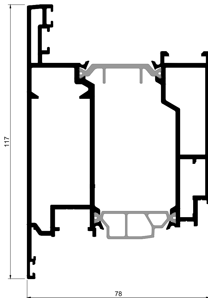
NST.23 Aro Móvel Abt. Exterior C16
