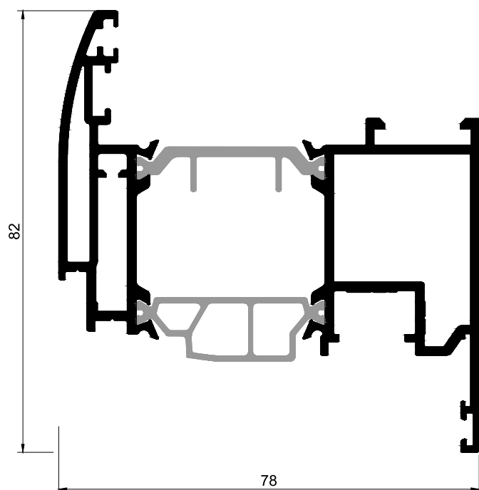
NST.08 Aro Móvel C16
