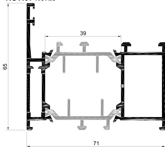
NST.07 Aro Fixo
