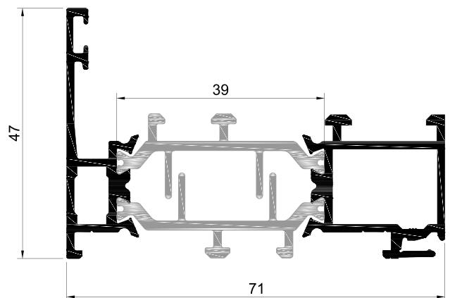
NST.41 Aro Fixo
