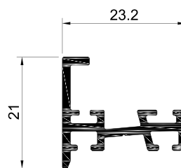
IT.33 Bite Inferior Vedação
