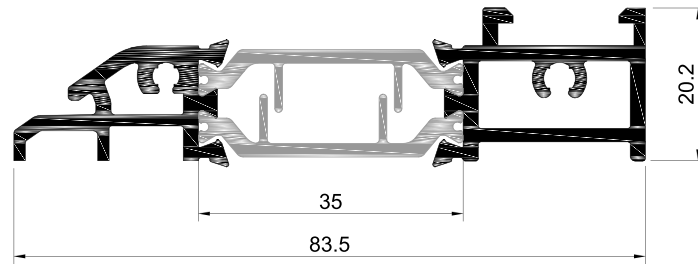
NST.49 Soleira Inferior
