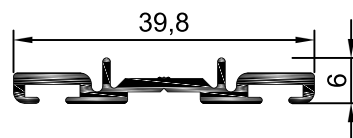
POC.27 Perfil Vedação
