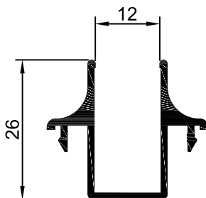
POC.84 Redutor P/ Lâminas Móveis
