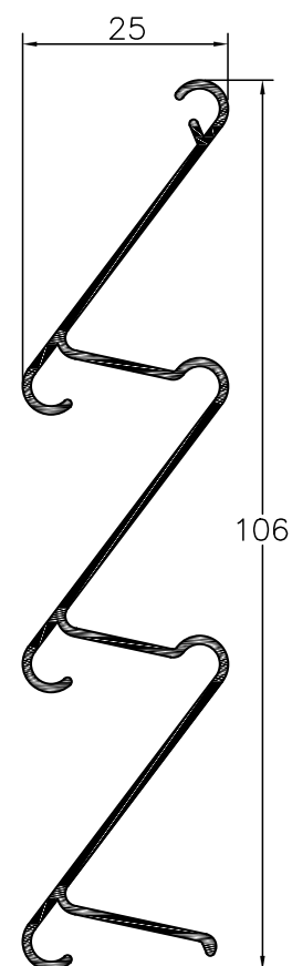
PO.38 Remate Lâmina
