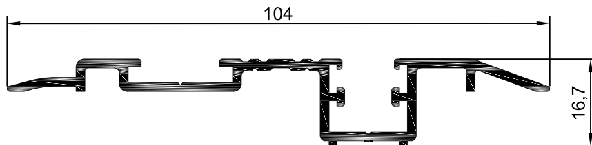
POC.42 Aro Fixo Inferior Harmónio (Soleira)
