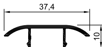
POC.14 Central Móvel
