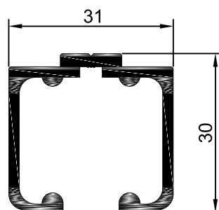
POC.63 Aro Fixo Superior Harmónio (Padeira)
